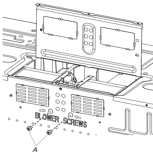
A. Tornillos del soplador (en orificios embutidos)
