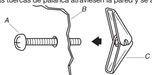
A. Perno de cabeza redonda de 3/16 -24 x 3" (7,6 cm) B. Placa de montaje C. Tuerca de palanca con resorte
