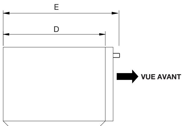
VUE LATÉRALE
